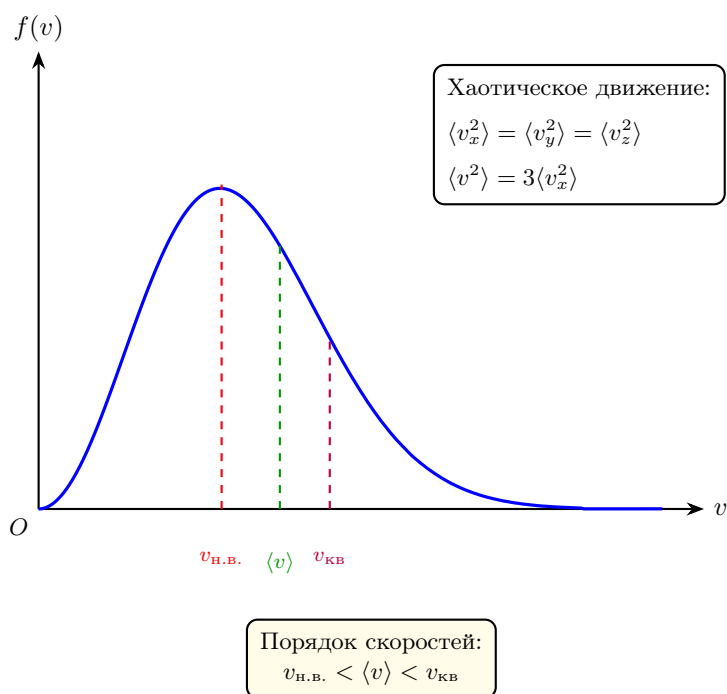
Рис. 32: Распределение Максвелла: не все молекулы имеют одинаковую скорость. Показаны наиболее вероятная v_{\text{н.в.}} , средняя \langle v \rangle и среднеквадратичная v_{\text{кв}} скорости.
