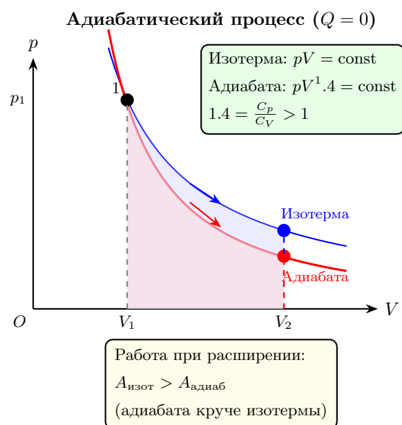
Рис. 35: Сравнение адиабатического и изотермического процессов на pV -диаграмме. Обе кривые начинаются в точке 1. Адиабата (красная) круче изотермы (синяя), поэтому при расширении от V_1 до V_2 работа газа в адиабатическом процессе меньше: A_{\text{адиаб}} < A_{\text{изот}} .
