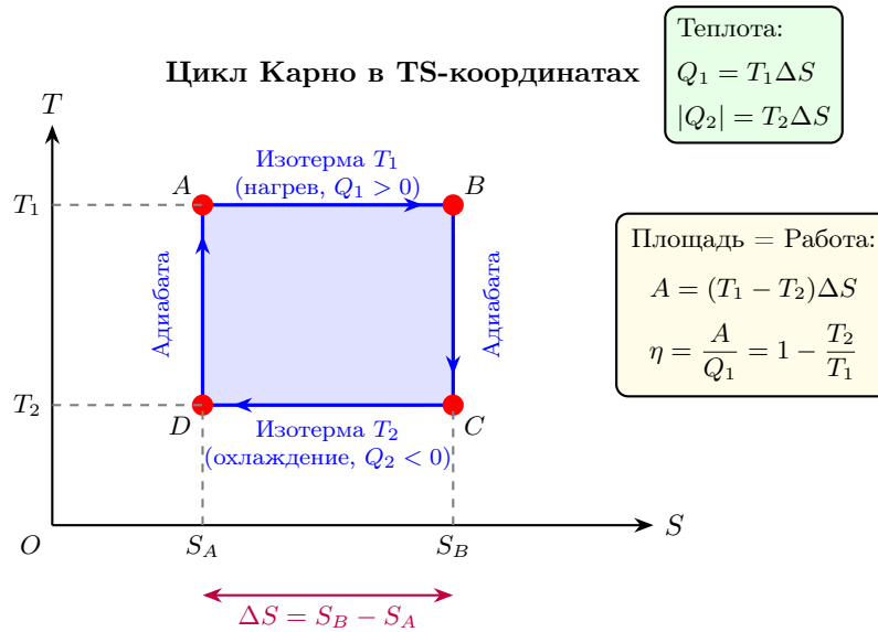
Рис. 38: Цикл Карно в TS-координатах. Прямоугольник ABCD : изотермы T_1 и T_2 (горизонтальные линии), адиабаты (вертикальные линии, S = \text{const} ). Площадь прямоугольника равна работе A = (T_1 - T_2)\Delta S . КПД цикла \eta = 1 - T_2/T_1 .
