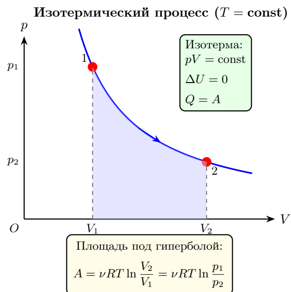
Рис. 34: Изотермический процесс на pV -диаграмме. Кривая — гипербола p = \nu RT/V . Работа газа равна площади под гиперболой между V_1 и V_2 (заштрихованная область).
